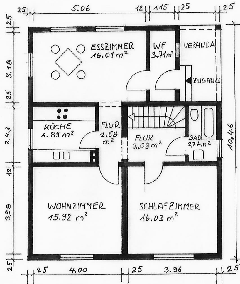
ERDGECHOSS
