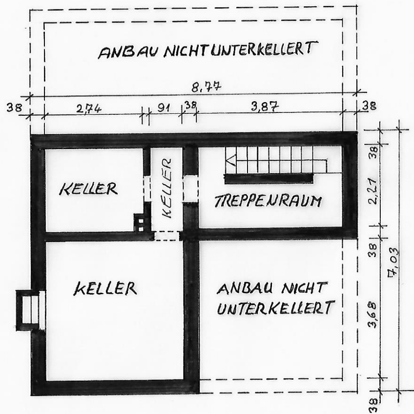
KELLERGECHOSS
